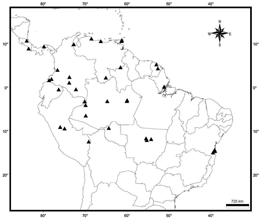
Fig. 2. – Distribution géographique de Gnamptogenys concinna dans la région Néotropicale.
